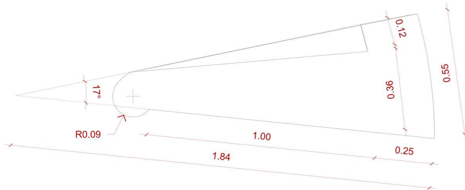
Κάτοψη
