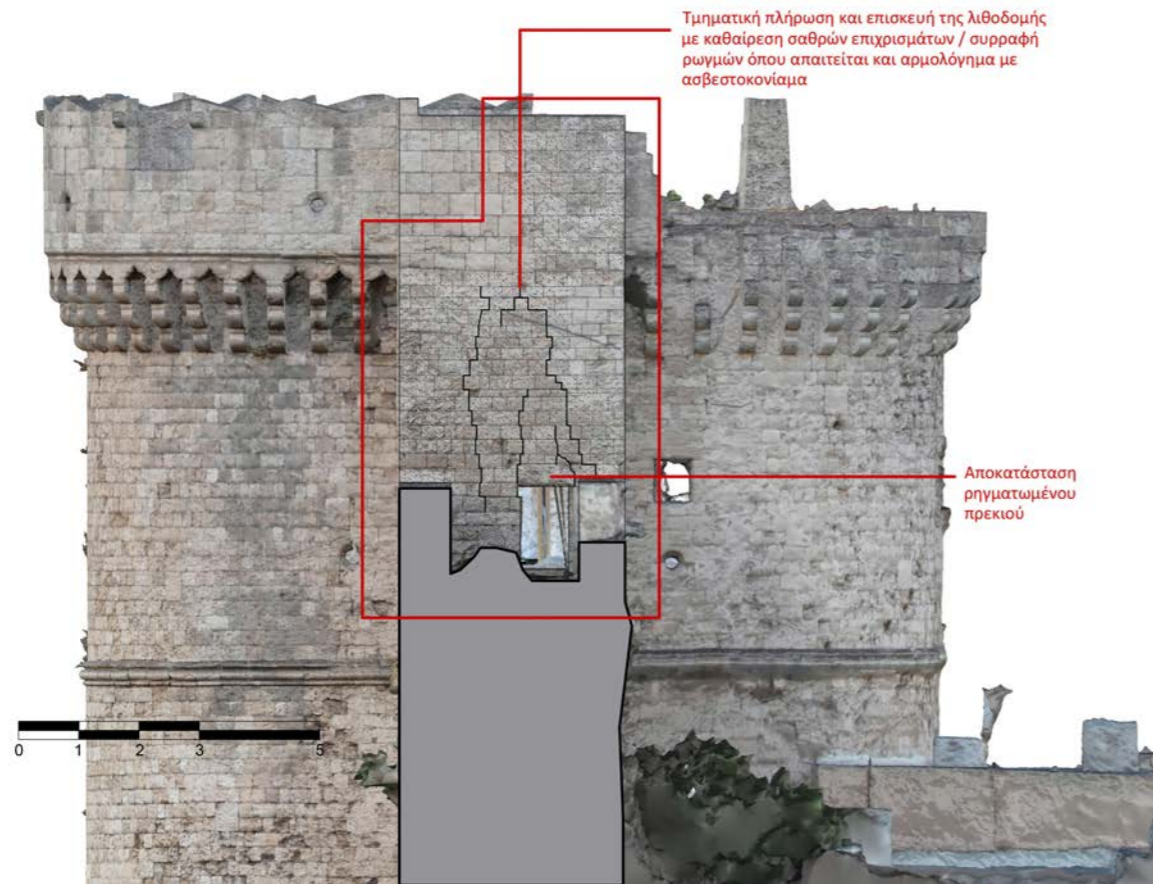
Εικ 12. Όψη Βόρειας Λιθοδομής
